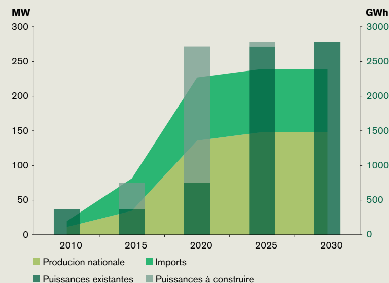
Figure 7 Puissances électriques et consommation
